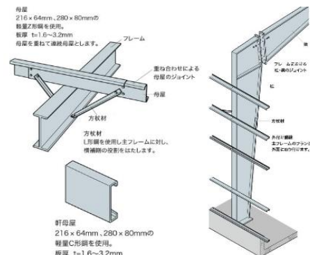
鉄骨詳細図
